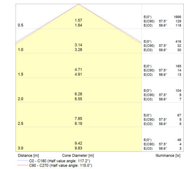
LVK Kegel
