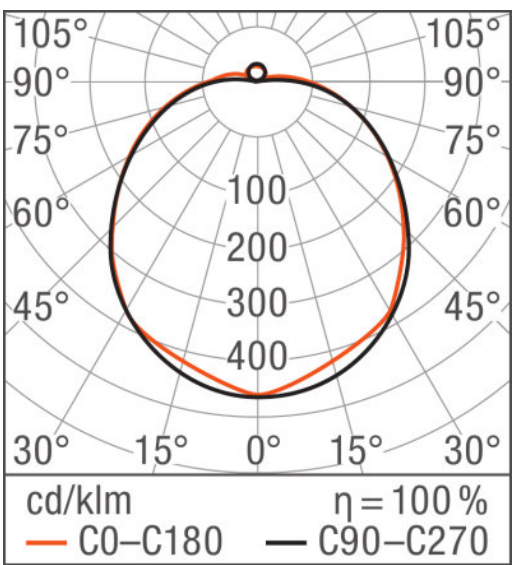
LVK Polar
